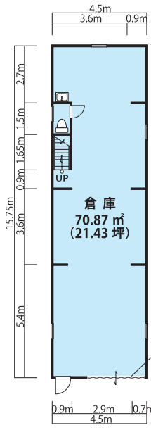
【1階平面図】
